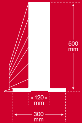
METON VI Stahl / Beton
